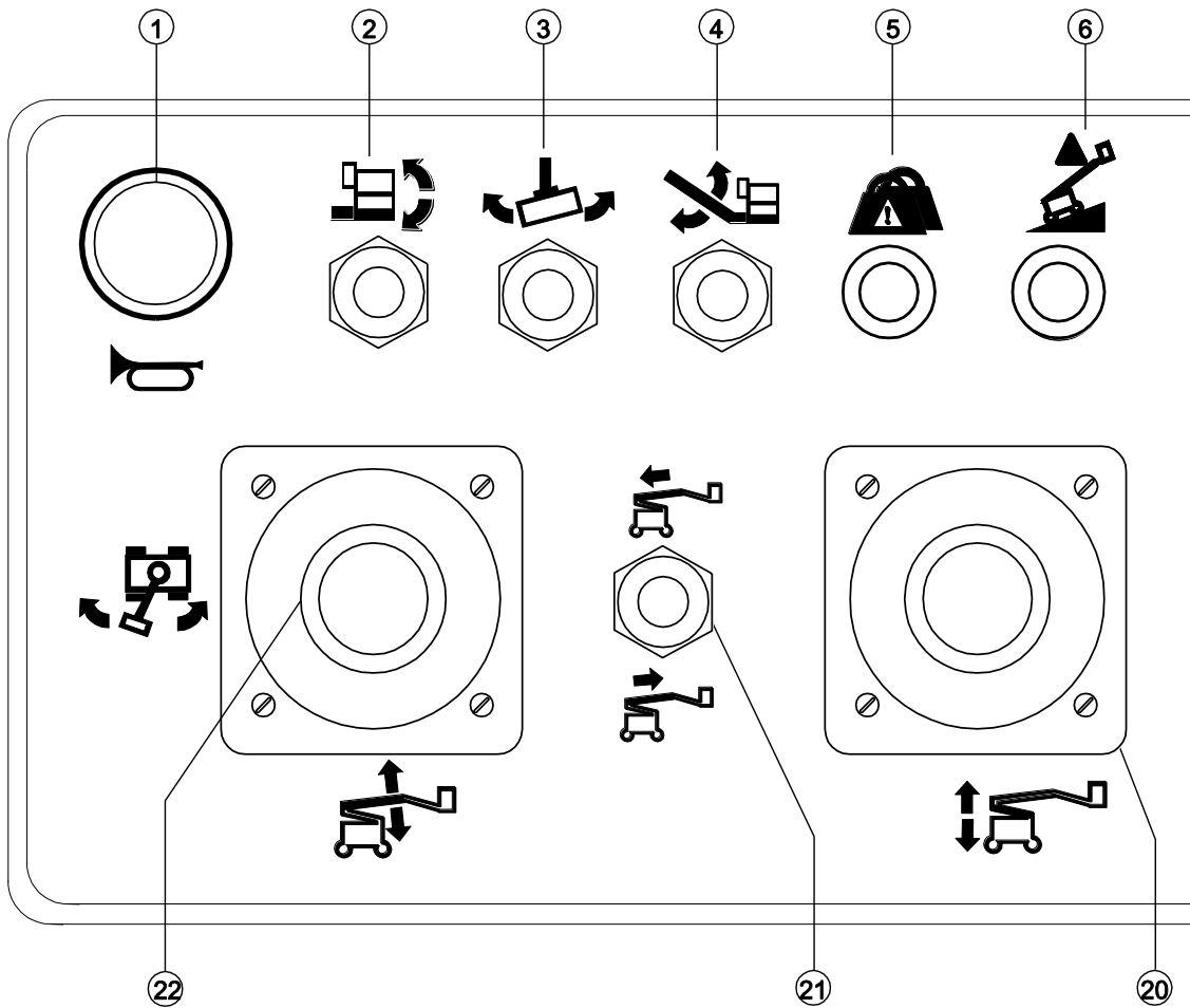
Plattformsteuerpult mit LCD-Display
