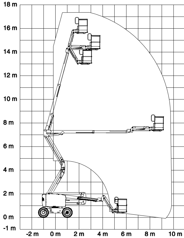
Reichweitentabelle Z-51/30J
