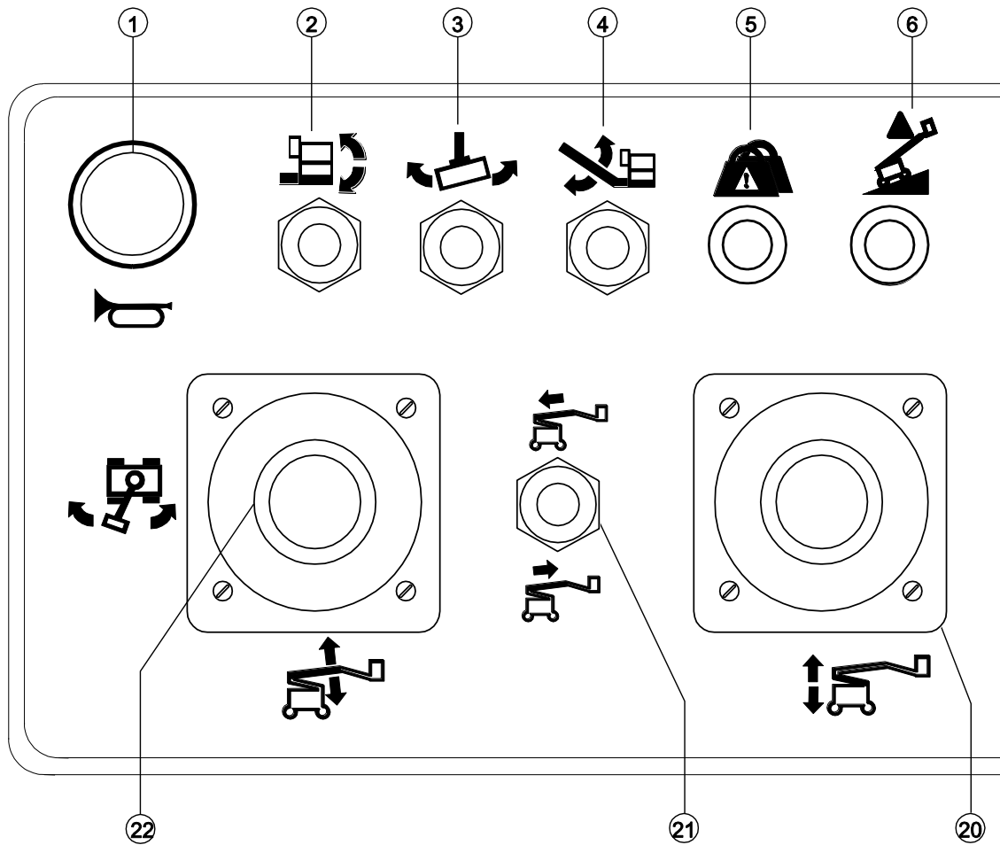
Plattformsteuerpult mit Betriebsstundenzähler
