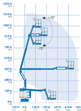
ARBEITSDIAGRAMM Z TM -34/22N
